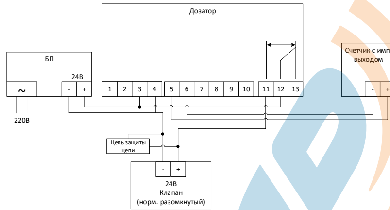
Рис.2 Схема подключения со счетчиком воды
