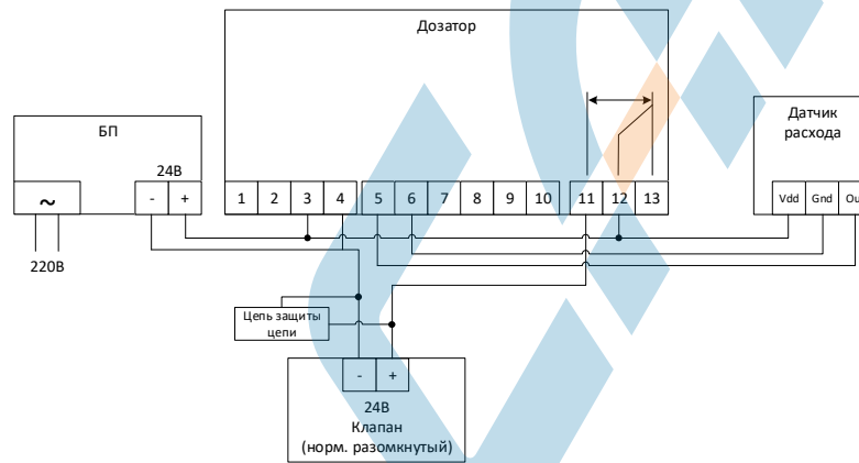
Рис.3 Схема подключения с датчиком расхода
