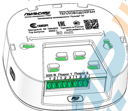
Рисунок 3 - Расположение разъемов и маркировки контактов на сигнализаторах
