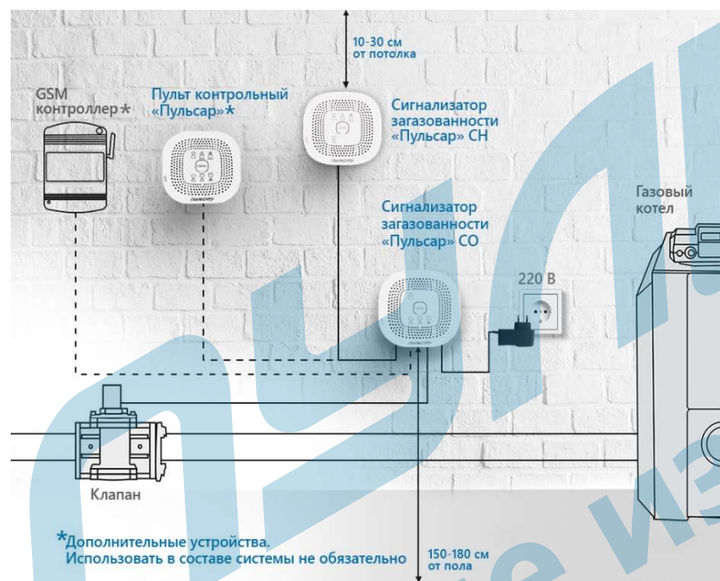
Рисунок 5 – Схема расположения компонентов системы автоматизированного контроля загазованности «Пульсар»
