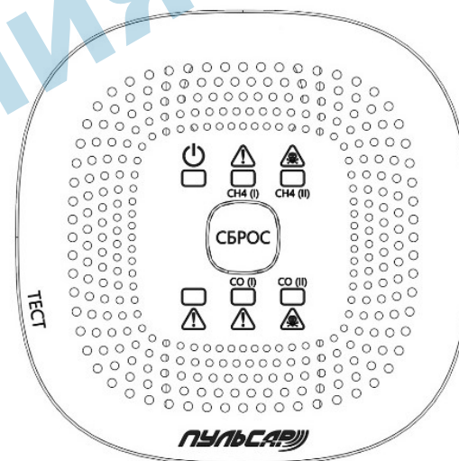
Рисунок 2 – Внешний вид пульта контрольного «Пульсар»
